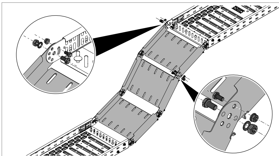
Jn. 72: Liigendpoogna elemendi paigaldamine
