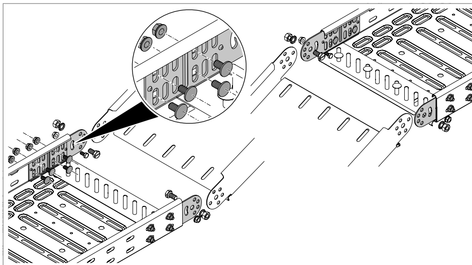
Jn. 71: Liigendjätke paigaldamine kaablirenni külge
