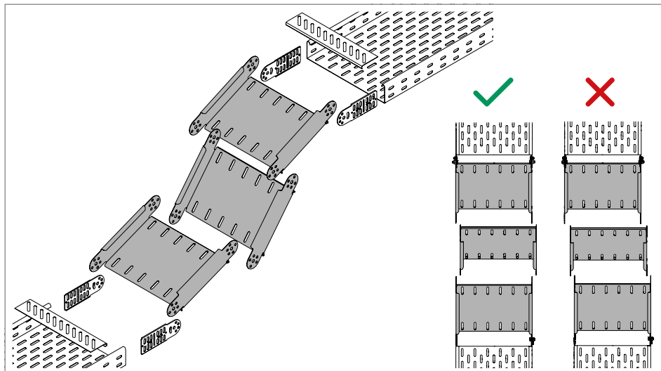
Jn. 69: Liigendpoogna element pooliku liigendjätku ning ülemineku- ja allaviiguplaadiga.
