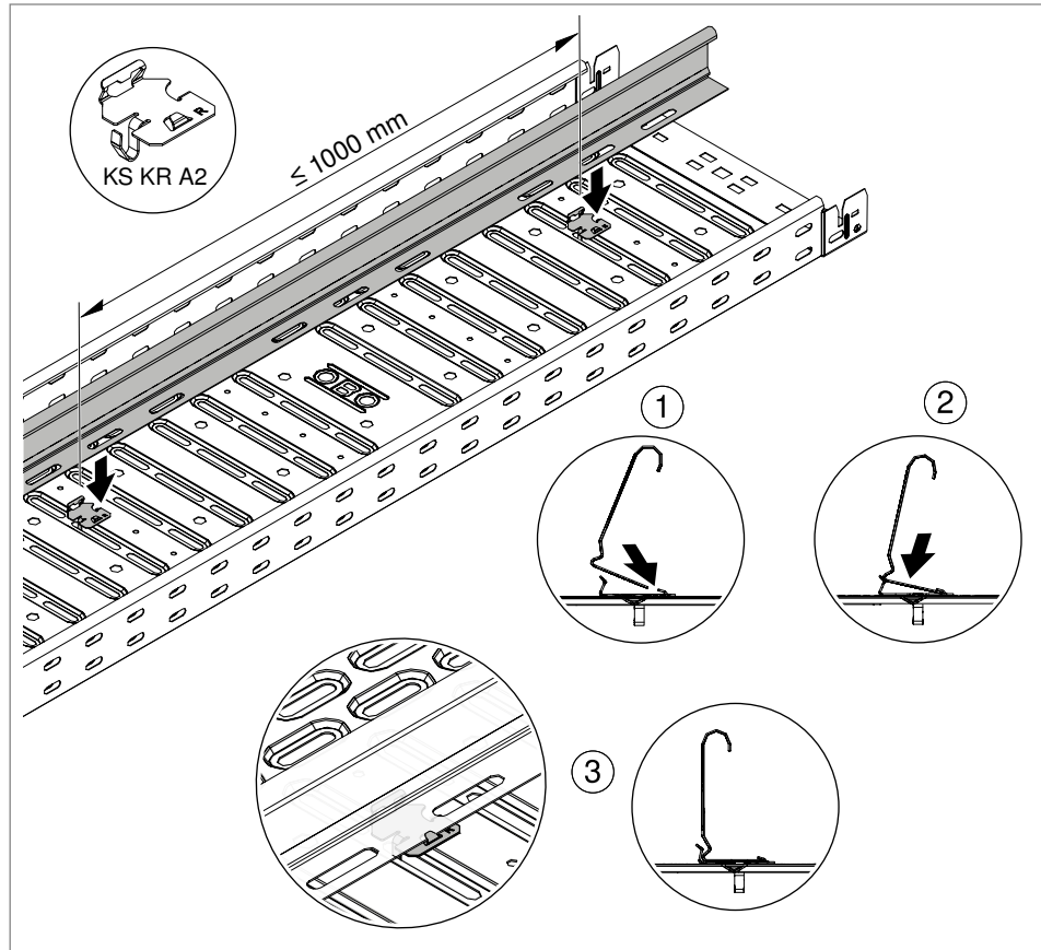
Jn. 80: Eraldusriiuli paigaldamine kinnitusklambrisse
