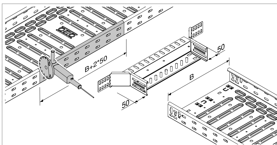
Jn. 55: Kaablirenni külje sälkamine
